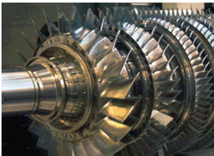
Versuchsverdichter
