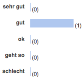
Abbildung 5: Statistik
